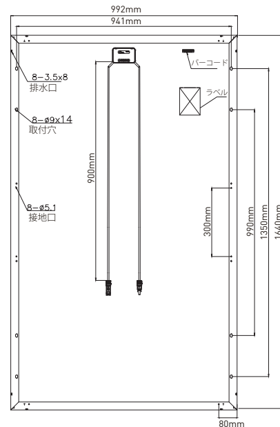
背面図
